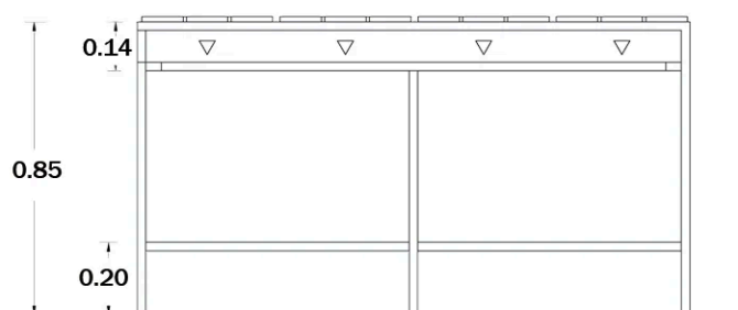
ALZADO FRONTAL
